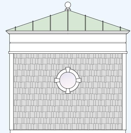
SIDE ELEVATION 10'L
